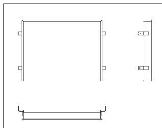
Marco remate obra de 3 lados (borde 3mm)
