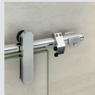
Detalle Soporte de Barra y Tope de Freno
