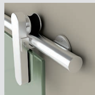
Detalle de rueda y antidescarrilamiento
