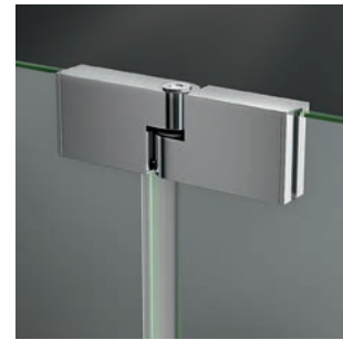
Detalle Bisagra Vidrio-Vidrio Polary
