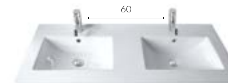
Double washbasin \varnothing 46,5 cm Doble poza \varnothing 46,5 cm Double vasques \varnothing 46,5 cm
