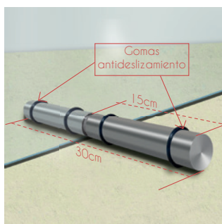
Detalle soporte grosor 25mm. Acero Inoxidable macizo.
