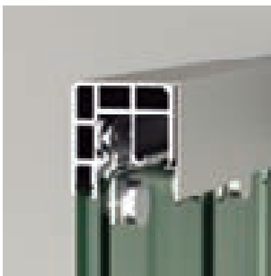
Detalle cerco superior. Modelo Cinebra 2P+F
