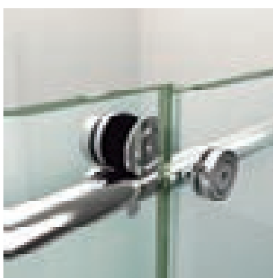
Detalle rodamiento y soporte de vidrio
