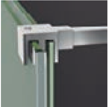
Detalle sujeción de barra superior
