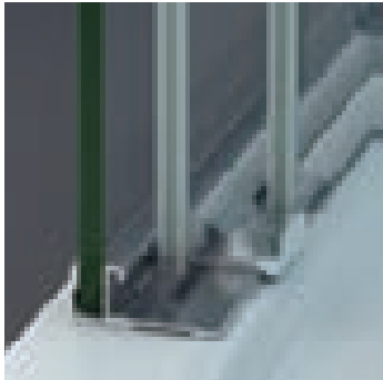
Detalle cerco inferior 2P+F. Vista interior
