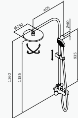
Columna Fija XL con desviador
