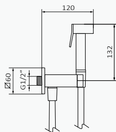
Intimixer 1 agua Quadro
