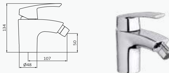
Bidé Monomando
