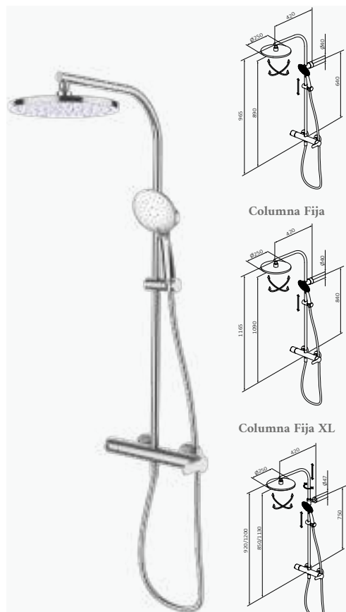
Columna Telescópica
