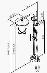
Columna Telescópica con desviador
