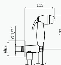
Intimixer 1 agua Hydrobrush
