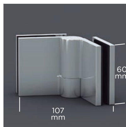
Detalle de bisagra plegable
