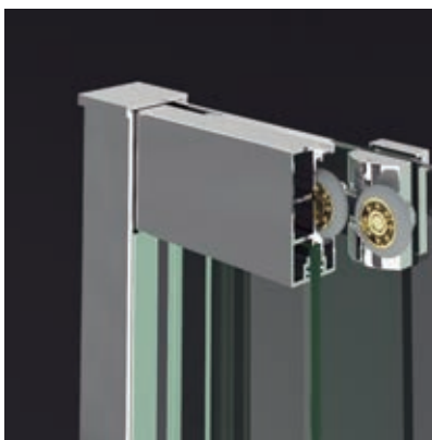
Detalle rodamiento superior
