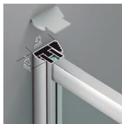
Detalle cerco compensador Riaza Enmarcada
