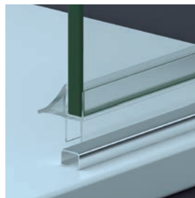
Detalle perfil de estanqueidad.
