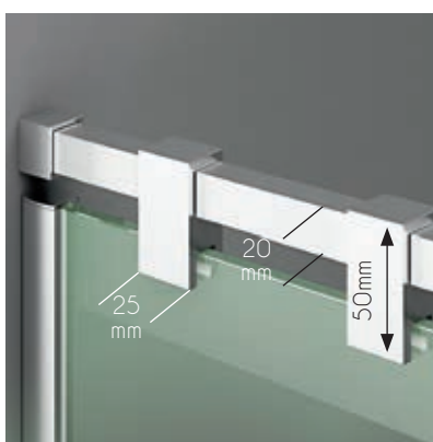
Detalle soporte de barra 180°
