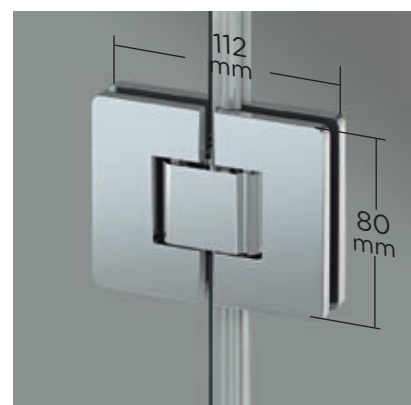
Detalle de bisagra vidrio-vidrio Aluminio-Zamak
