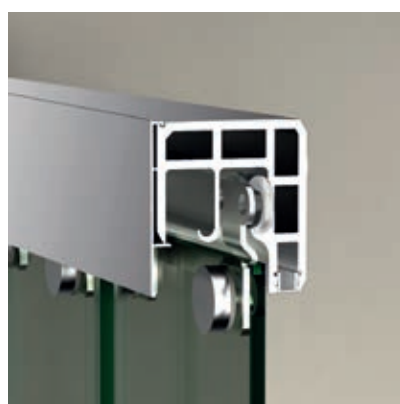
Detalle cerco superior 2P Vista interior
