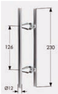
Detalle tirador Semicircular
