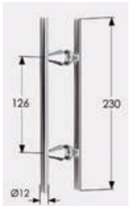
Detalle tirador Semicircular
