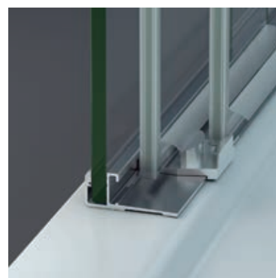
Detalle cerco inferior 2P+F Vista interior
