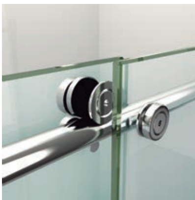
Detalle rodamiento y soporte de vidrio
