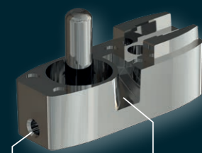
Fijación para alinear la puerta Sistema de desaguado del pivote inferior
