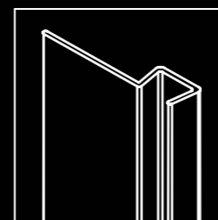
Junta cruce de vidrios 18mm | 6 mm
