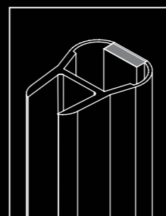
Junta magnética plana 180°. Cajetín 12 mm 6/8 mm
