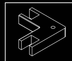
Esquinero inferior perfil vierteaguas metálico
