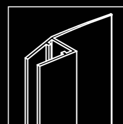
Junta de ala 18 mm para abatible. Cajetín 12 mm | 6/8 mm
