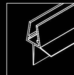
Junta vierteaguas inferior ala 19 mm 6/8mm
