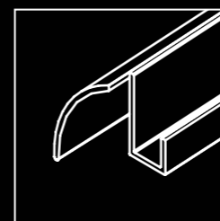
Junta vierteaguas inferior puerta 6 mm
